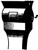
Fig. 36. Winkelgelenk der Technik. 1 Achse. 2 Pfanne. 3 Die cylindrische Rolle. 4 Der Zapfen.
